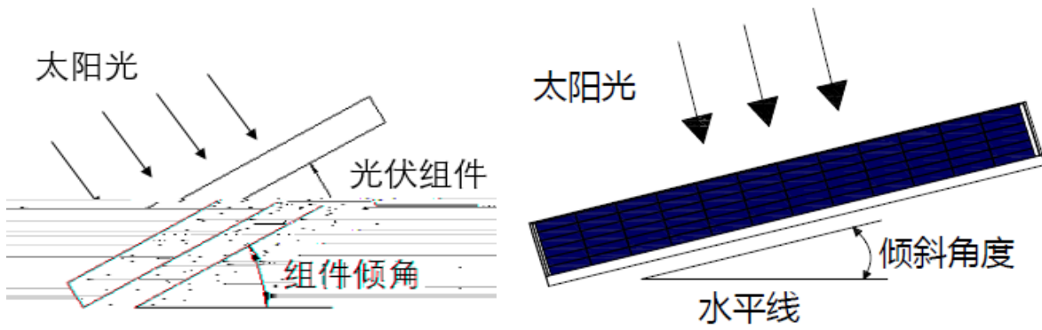
图 1 组件安装的角度
